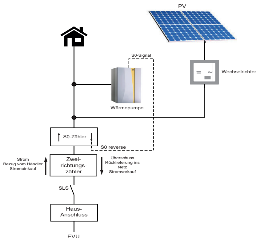
Einbindung S0-Signal / Überschuss
