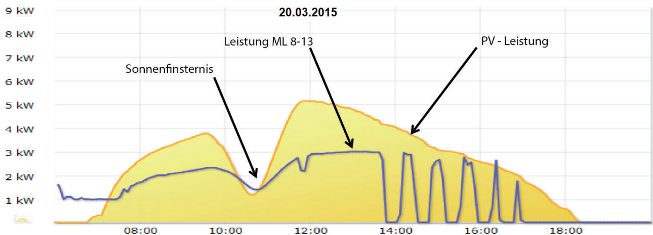
Momentanleistung der PV-Anlage / Leistungsaufnahme TERRA ML 8-13
