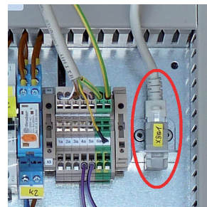
Netzbuchse im Inneren einer AERO ILM Wärmepumpe an der Elektrik
