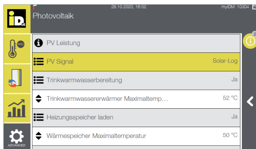
Einstellung PV-Signal „Solar-Log“ Navigatorregelung
