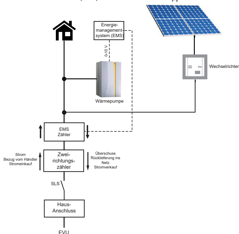
Einbindung 0-10V Signal / Überschuss
