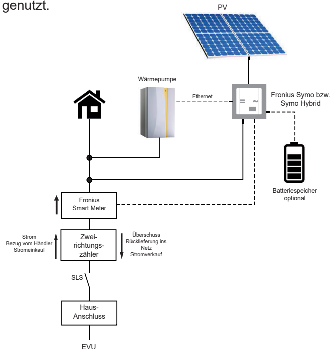
Einbindung Fronius Wechselrichter
